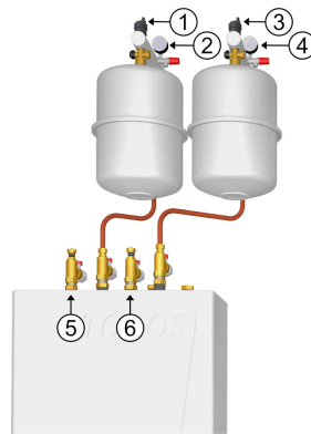
Figuur 13 Onderdelen t.b.v. ontluchten en vullen bron of cv-systeem
