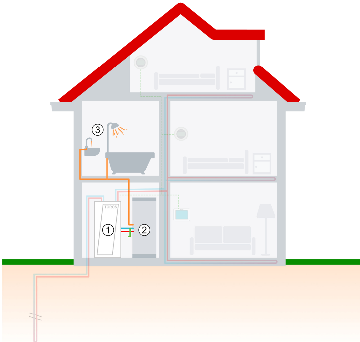
Figuur 6 Schematische weergave van de tapwaterinstallatie 1: Warmtepomp 2: Boilervat 3: Warm tapwater (kranen en douche/bad)
