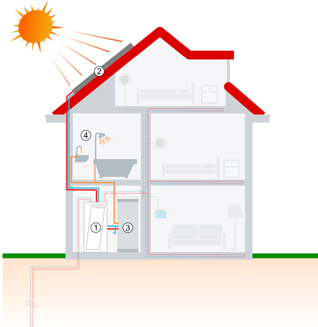
Figuur 7 Schematische weergave van een installatie met zonnecollectoren
