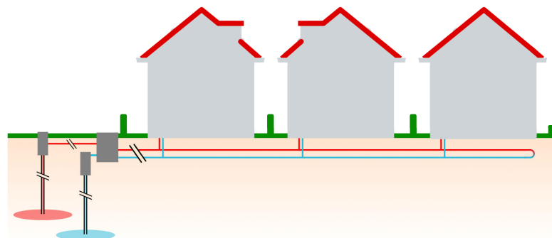
Figuur 3 Schematische weergave van een collectieve open bron
