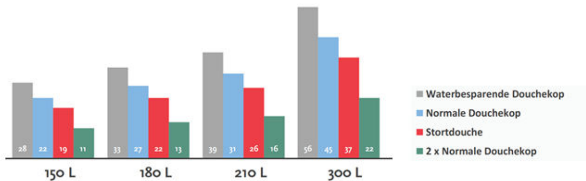
Figuur 12 Indicatieve douchetijd in minuten bij verschillende boilervatformaten en douchekoptypes
