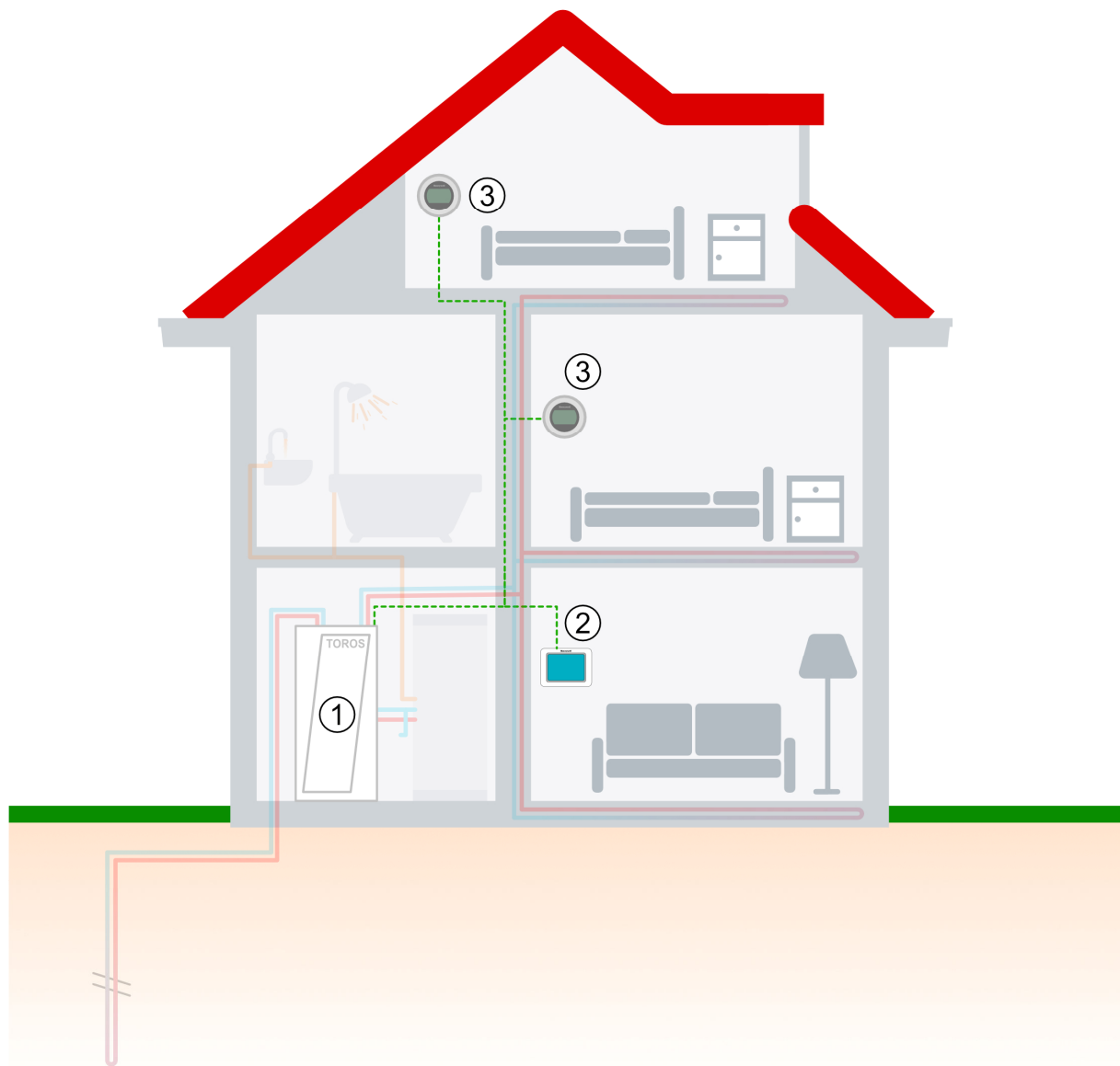
Figuur 5 Diverse thermostaten door de woning 1: Warmtepomp 2: Hoofdthermostaat 3: Secundaire thermostaten
