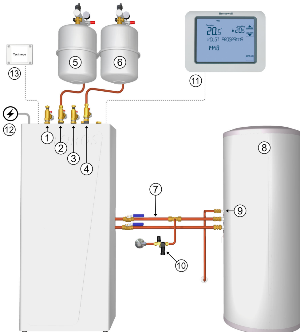
Figuur 8 Onderdelen van de warmtepompinstallatie
