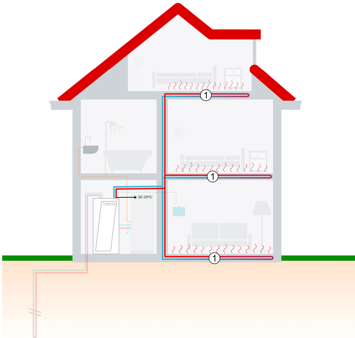
Figuur 4 Vloerverwarming door de gehele woning met een aanvoertemperatuur rond 30-35 graden
