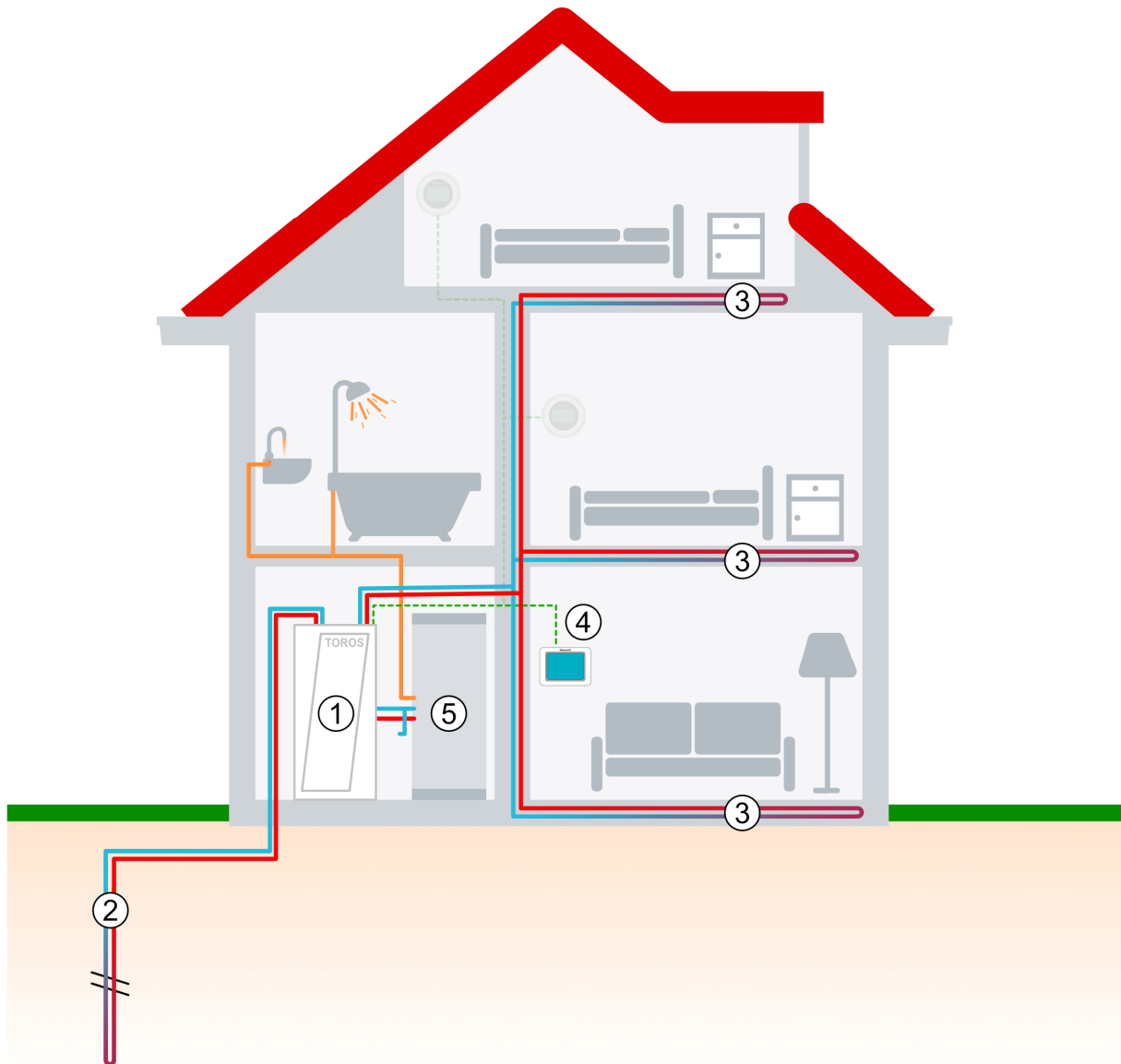
Figuur 1 Schematische weergave van warmtepompinstallatie
